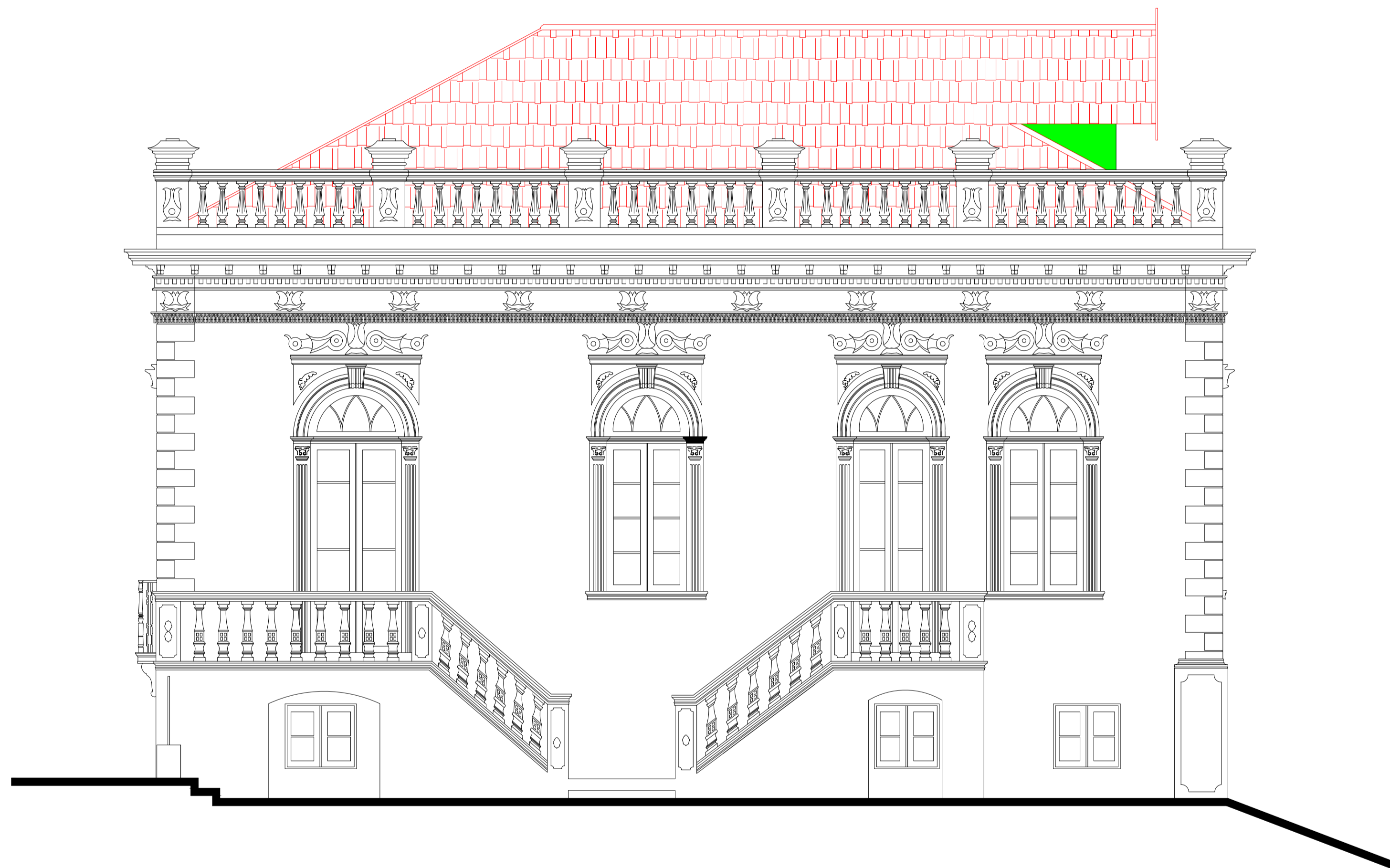
VISTA 03 ESC.: 1/50
