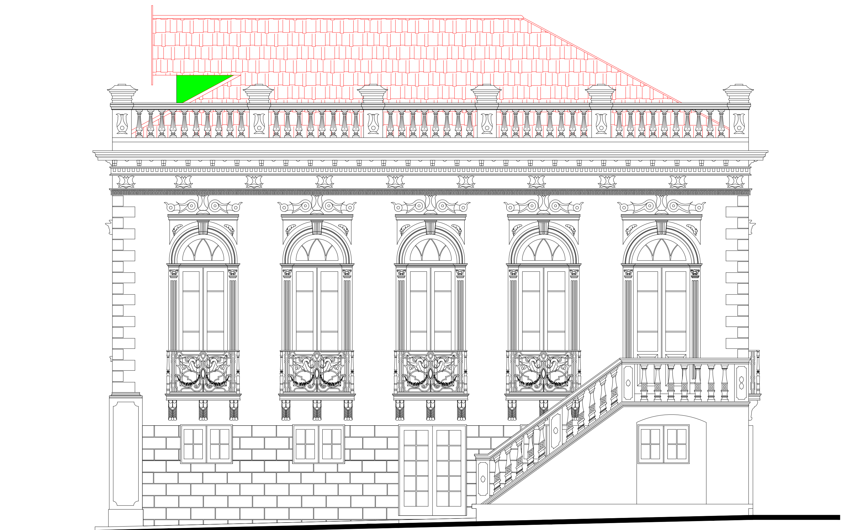
VISTA 01 ESC.: 1/50
