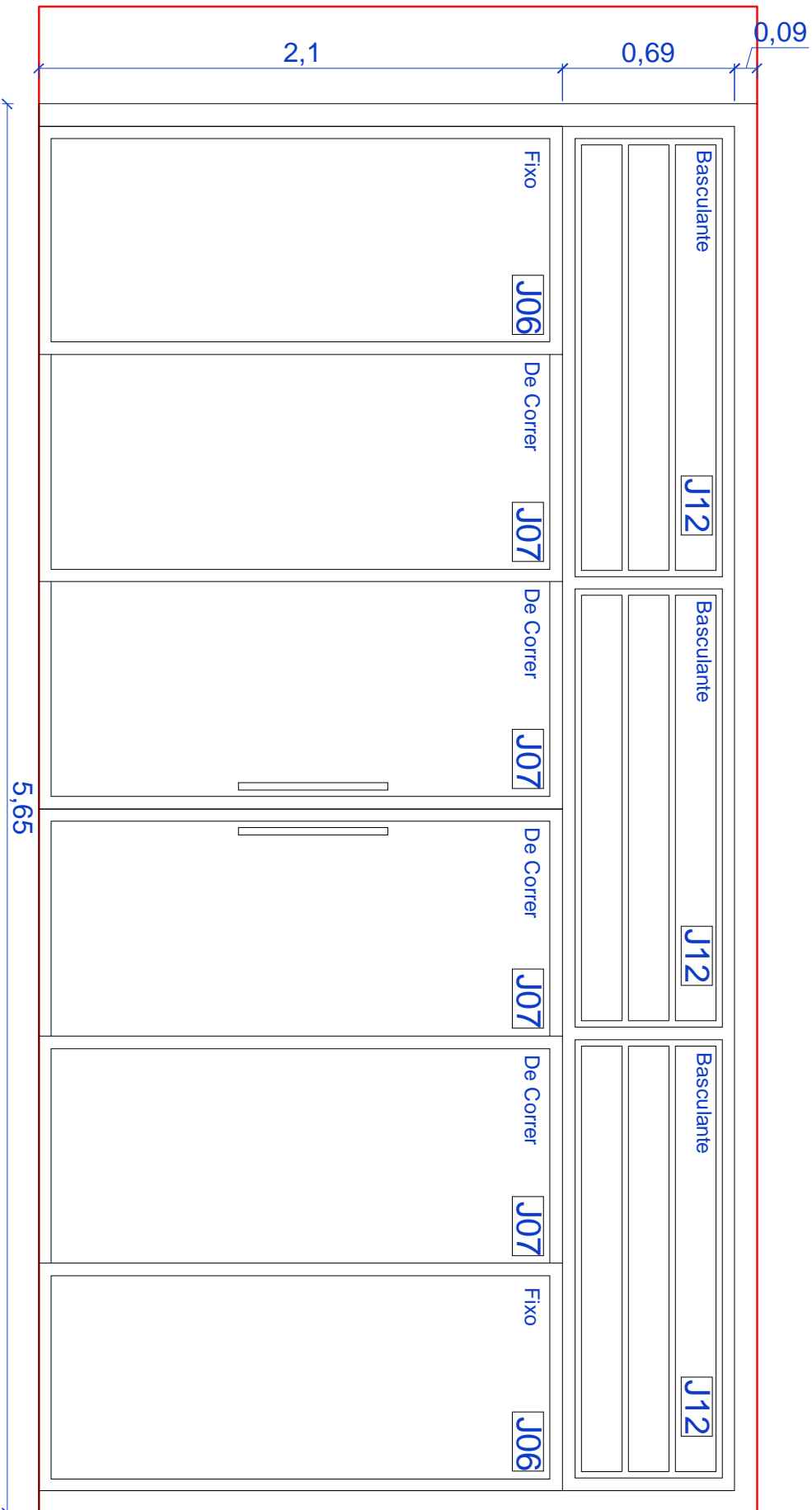
Vista 02 Esc.: 1/20
