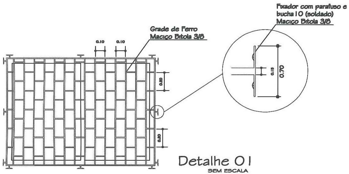
Grade Interna para Janela SEM ESCALA
