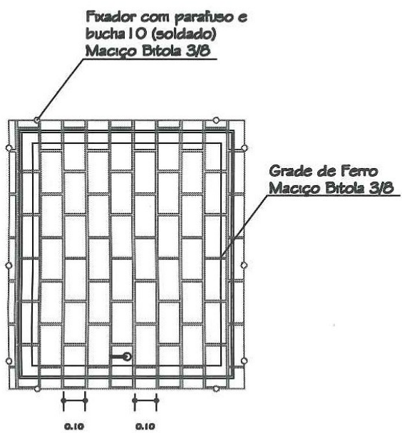
Grade Externa para Janela SEM ESCALA
