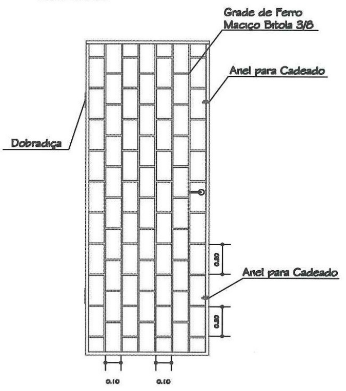
Porta Externa de Ferro SEM ESCALA
